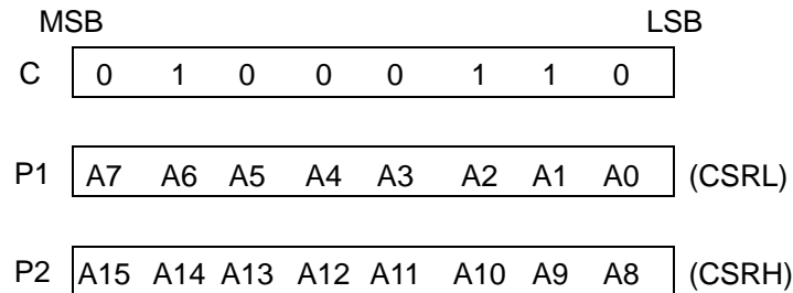
Fig.37 CSRW parameters
