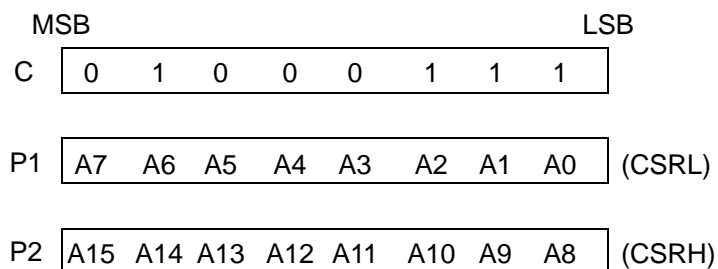
Fig.38 CSRR parameters
